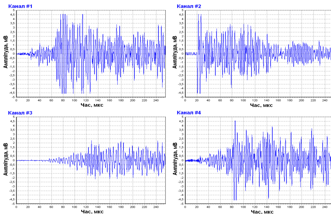
Рисунок 2 – Хвильове відображення сигналів АЕ, збуджених одним джерелом, зареєстровані вимірвальними каналами
