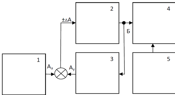
Рисунок 2 – Схема компенсації похибки у пропонуваному методі для окремого акселерометра МСК
