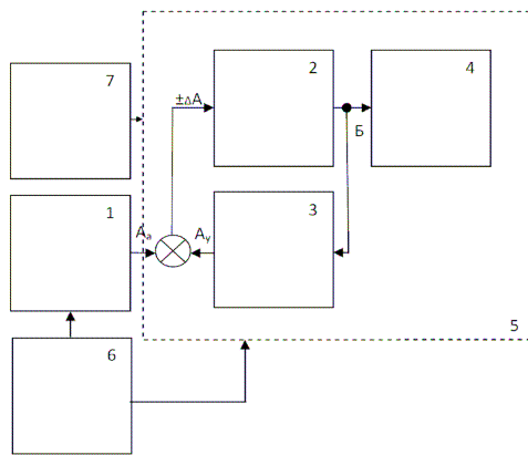
Рисунок 3 – Схема компенсації завдан в пропонуваному пристрої для окремого акселерометра МСК
