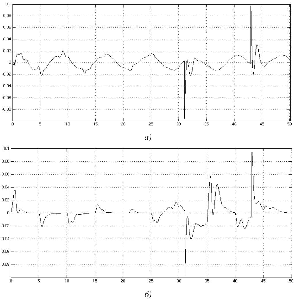
Рисунок 6 – Відхилення регульованої величини від вихідної величини еталона при подачі на вхід системи сигналів у вигляді гладких (а) та стрибкоподібних (б) функцій
