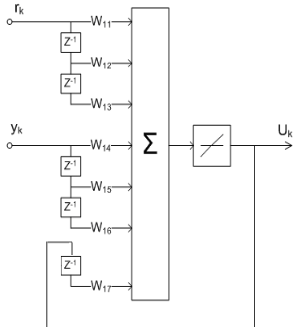
Рисунок 3 – Структурна схема нейронного ПД-контролера
