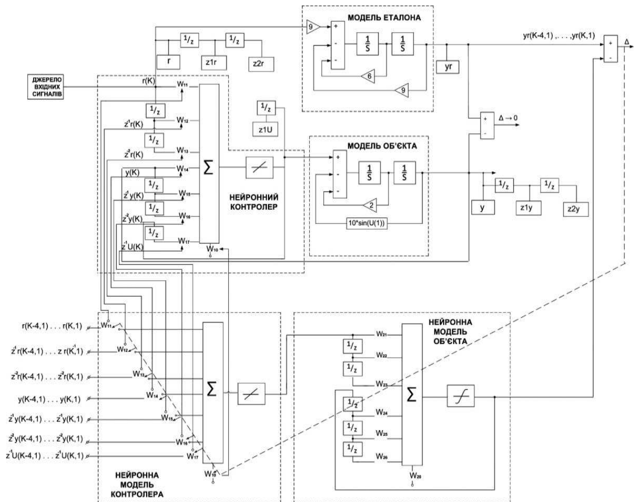
Рисунок 4 – Узагальнена схема адаптивного навчання нейронної моделі ПД-контролера при використанні функції train
