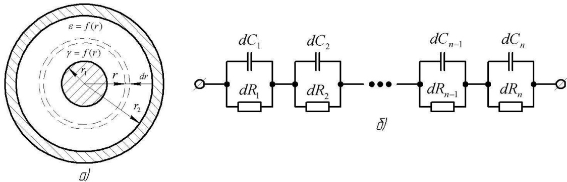
Рисунок 1 – Поперечний переріз (а) і диференціальна схема заміщення електричної ізоляції (б) коаксіального кабеля
