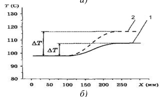
Рисунок 2 - Схематичне зображення різновисхідної однорідної пластини (а) та розподілення температури на поверхні(б) при h = 0,9d (1) та h = 0,7d (2)
