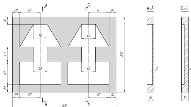
Рисунок 4 - Схематичне зображення зразка із штучними дефектами складної геометричної форми
