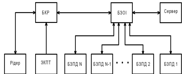
Рисунок 9 – Структурна схема інформаційно-вимірювальної системи контролю зоотехнічних параметрів тварин з системою радіочастотної ідентифікації на основі централізованого рідера великого радіусу дії та засобу контролю проходження тварини
