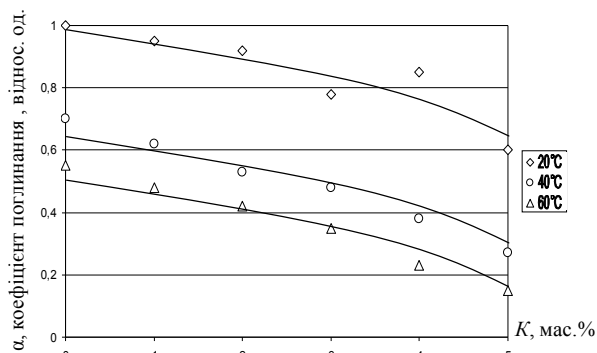
Рисунок 6 – Залежність коефіцієнта поглинання ультразвуку від концентрації палива в моторній оливі при температурах зразків 20, 40, 60 °С
