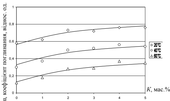
Рисунок 5 – Залежність коефіцієнта поглинання ультразвуку від концентрації води в моторній оливі при температурах зразків 20, 40, 60 °С
