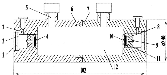
1, 8 – гайки; 2, 11 – фторопластові прокладки; 3 – кабельний канал; 4, 10 – випромінюючий та приймаючий ультразвуковий перетворювач, відповідно; 5 – отвір для заливання оливи; 6, 7 – два стикових корпуси; 8 – гайка; 9 – латунні вставки; 12 – вимірювальна камера
