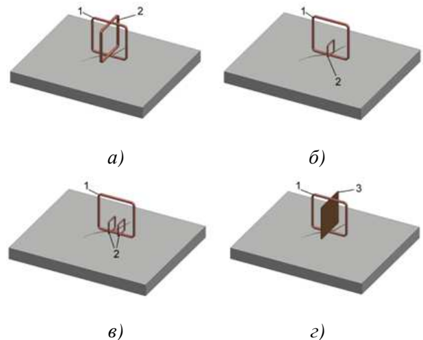
1 – возбуждающая обмотка; 2 – измерительная обмотка; 3 – электропроводящая пластина
