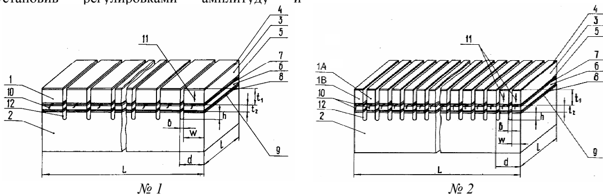
1 – пьезоэлементы; 2 – токопроводящий демпфер (вольфрам-фенопласт); 3 – пьезокерамика (цирконат-титанат-свинца); 4, 5 – металлические электроды; 6 – изолятор (оксид алюминия); 7, 8, 9 – металлические пленки; 10 – проводники для индивидуальных пьезоэлементов 1, для попарного электрического объединения пьезоэлементов (1А, 1В) и для возбуждения/приема акустических/электрических колебаний; 11 – направление вектора поляризации пьезоэлементов; 12 – пазы между элементами решетки
