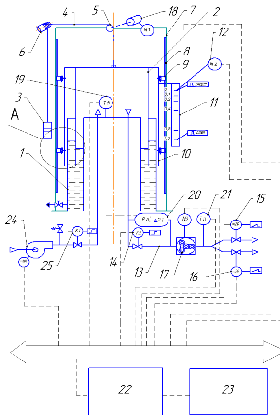
Рисунок 1 – Принципова схема удосконаленого еталона об'єму та об'ємної витрати газу дзвонового типу
