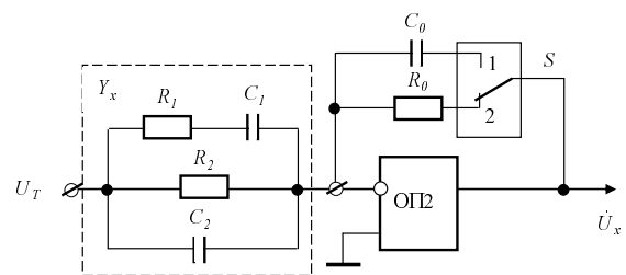
Рисунок 1 – Схема векторного перетворювача «імітанс-напруга»
