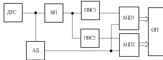
Рисунок 2 – Структурна схема засобу вимірювання параметрів чотириелементного двополосника
