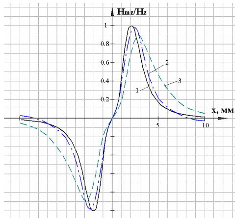
1 – експеримент; 2 – расчет по разработанной программе; 3 – расчет по упрощенной формуле
