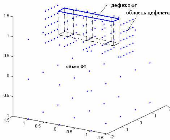
Рисунок 2 – Центры ЭО ФТ, содержащего дефект
