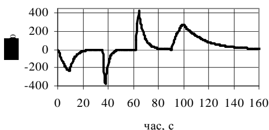
Рисунок 8 – Залежність відхилення частоти обертання турбіни в нестационарному режимі вимірювання \omega від частоти обертання \omega_0 , одержаної на базі градувальної кривої (рис. 3) за умов вибраної в часі (рис. 5) залежності зміни витрати газу на вході лічильника
