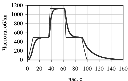
Рисунок 7 – Зміна частоти обертання турбіни для симетричної залежності зміни витрати (рис. 6) з урахуванням сил інерції (товста лінія) і без їх урахування (тонка лінія)
