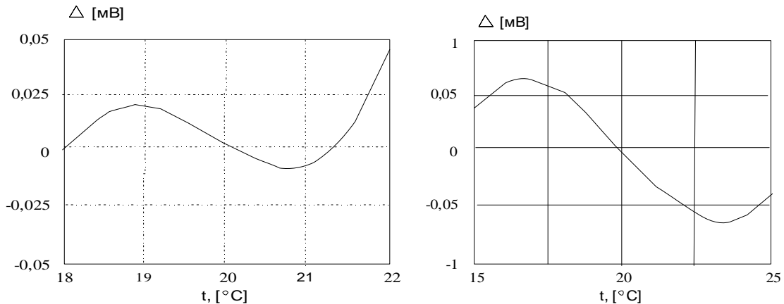
Рисунок 4 – Графічні залежності абсолютної похибки відтворення компенсаційної напруги
