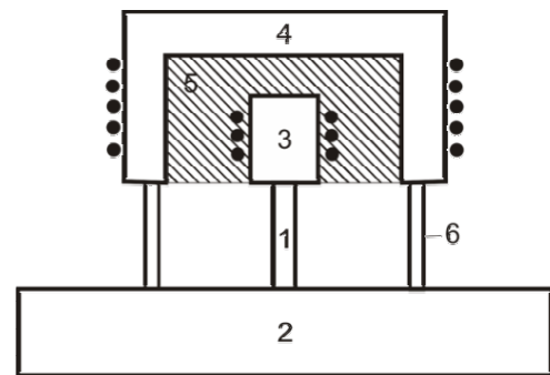
Рисунок 1 – Блок-схема вимірної комірки
