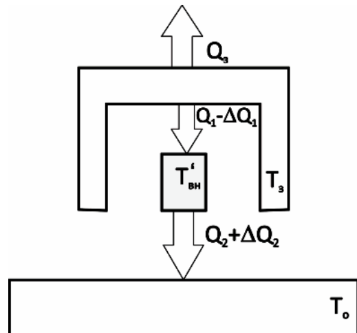
Рисунок 3 – Розподіл потоків тепла після ввімкнення внутрішнього нагрівника
