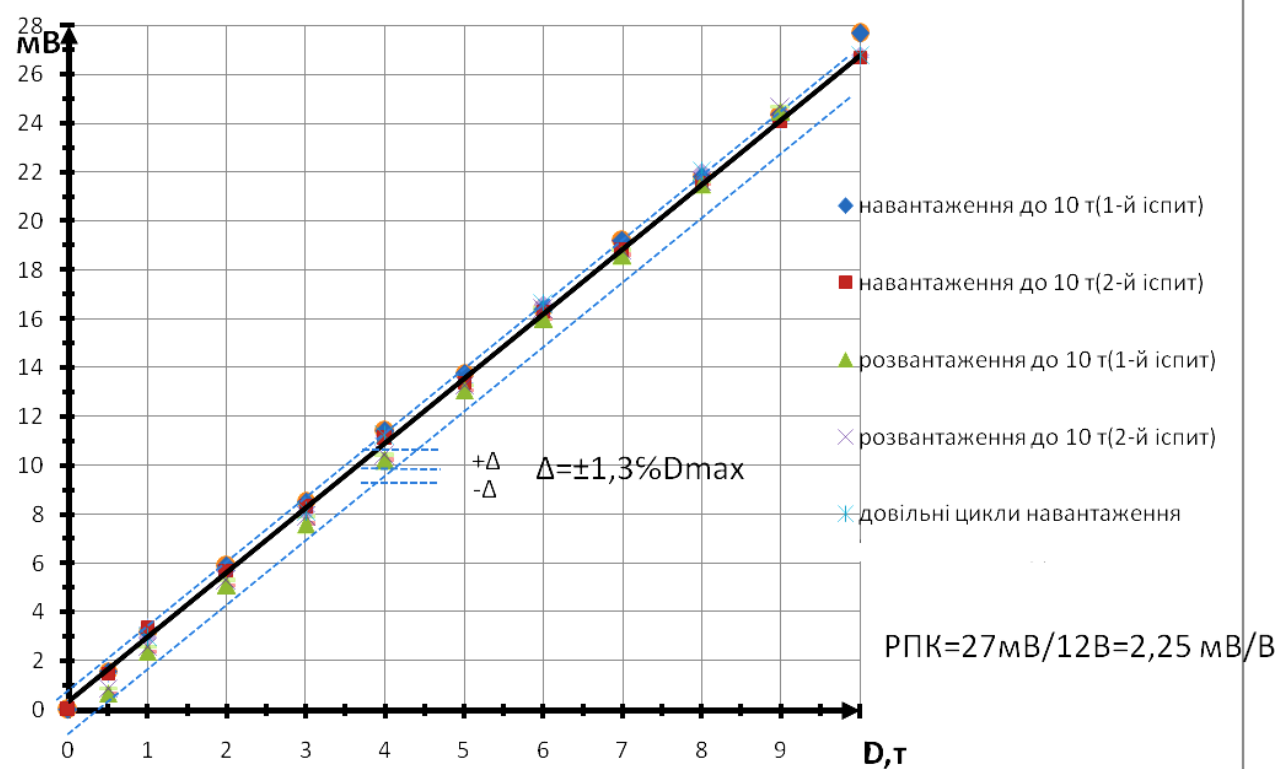
Рисунок 6 – Градувальна характеристика експериментального зразка давача 4201 ДСТ – 10
