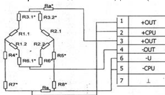
Рисунок 1 – Принципова електрична схема давача 4201 ДСТ - 10
